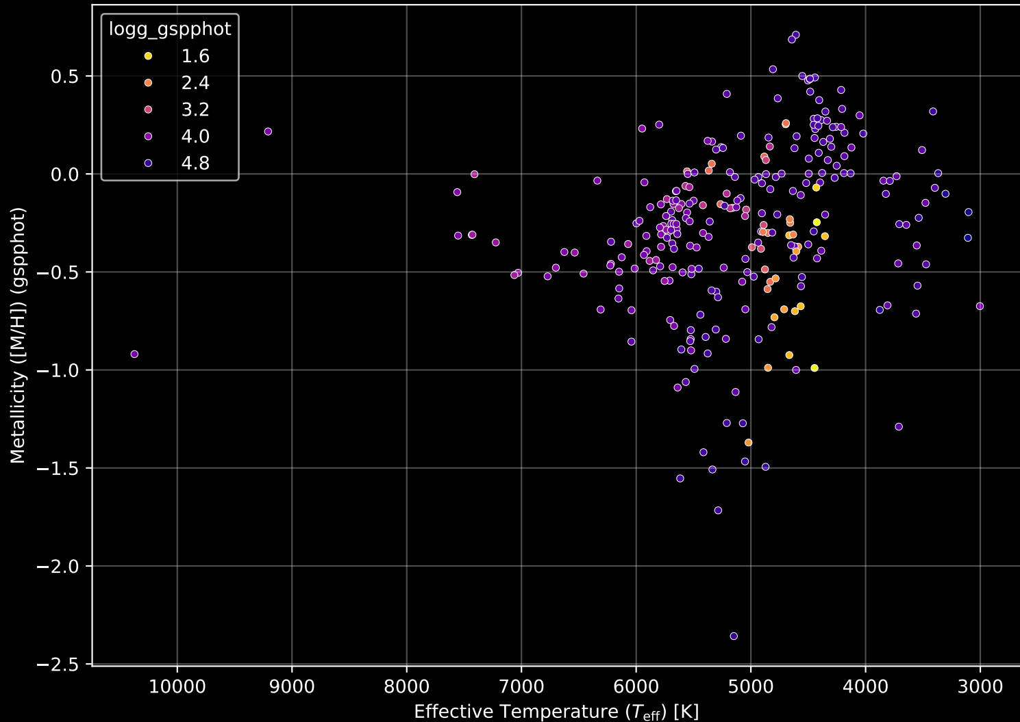
APOGEE DR17 Field: [M33] Stellar Population Parameters (n= 275)
